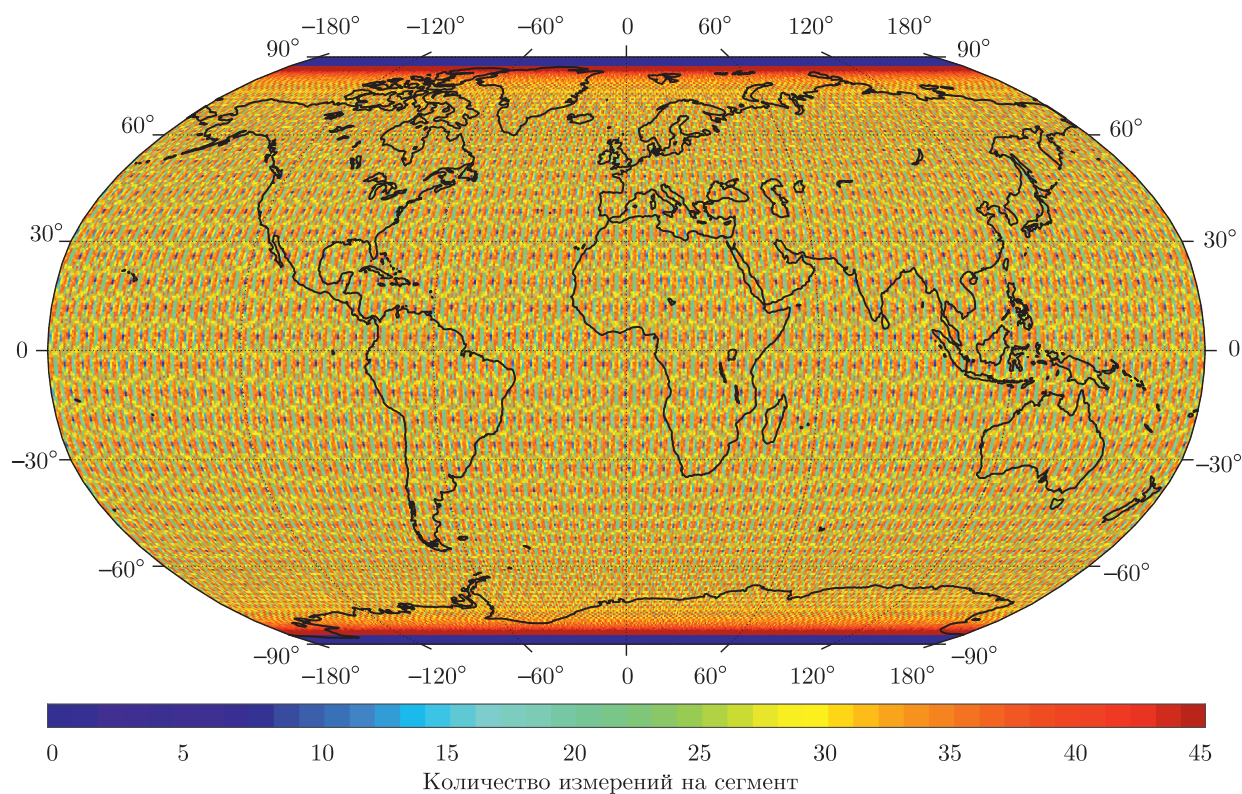
Рис. 8. (В цвете онлайн) Гистограмма покрытия поверхности Земли измерениями спутником с параметрами h = 224 \text{ км} , i = 96.7^\circ в сегментах 0.64^\circ \times 0.64^\circ на временном интервале 111 сут. Величина глобального покрытия 93.1 %
