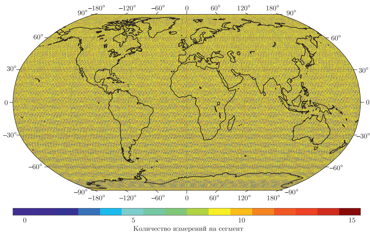
Рис. 4. (В цвете онлайн) Гистограмма покрытия поверхности Земли подспутниковыми трассами КА на орбите с параметрами h = 225 км, i = 89.9^\circ в сегментах 0.3^\circ \times 0.3^\circ на временном интервале 147 сут (величина глобального покрытия 100 %)
