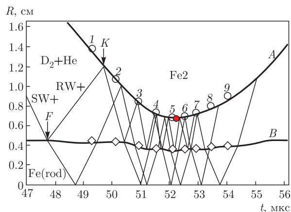
Рис. 6. (В цвете онлайн) Сравнение экспериментальных и рассчитанных R(t) -данных в опыте М10 со смесью дейтерия и гелия. Обозначения, как на рис. 5
