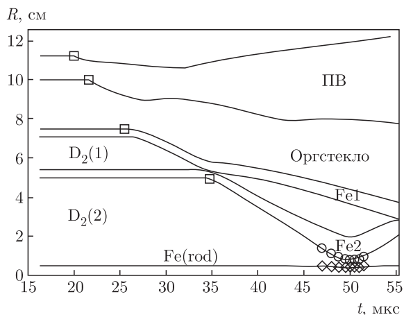
Рис. 4. Экспериментальные данные и рассчитанные R(t) -диаграммы. Эксперимент: квадраты — электроконтактная методика; кружки — внутренняя граница оболочки второго каскада Fe2 (ВГО2); ромбы — граница стального стержня Fe(rod), ПВ — продукты взрыва. Сплошные линии — расчет, в области дейтерия использовано УРС из работы [26]
