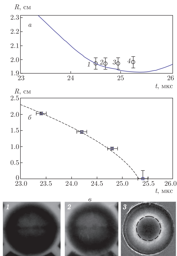
Рис. 10. а) R(t) -диаграммы движения внутренней границы оболочки в экспериментальном устройстве для измерения сжимаемости водорода в состоянии КЗ: значки — эксперименты [3]; кривая — расчет по УРС водорода [26]. б) Движение внутренней границы оболочки без газа: значки — эксперименты, штрихи — расчет. в) Рентгенограммы 1 и 2 из работы [3] соответствуют точкам 1 и 2 на рис. а; 3 — изображение сферической оболочки с использованием современной техники (штрихи — граница газ-металл)
