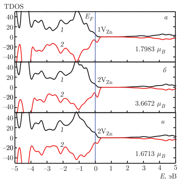
Рис. 4. Полная плотность состояний сверхрешетки (total density of states, TDOS) для случаев, когда спины направлены вверх (кривые 1) и вниз (кривые 2): а — с одной вакансией цинка V_{Zn} ; б — с двумя изолированными вакансиями цинка; в — с двумя близко расположенными вакансиями цинка
