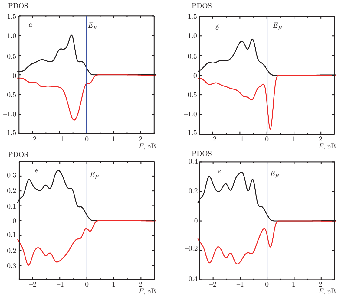
Рис. 7. Частичные электронные плотности состояний (partial DOS, PDOS): а — 2p-электрон атома O-I; б — 2p-электрон атома O-II; в — 3d-электрон атома цинка, связанного с атомом O-I; г — 3d-электрон атома цинка, связанного с атомом O-II
