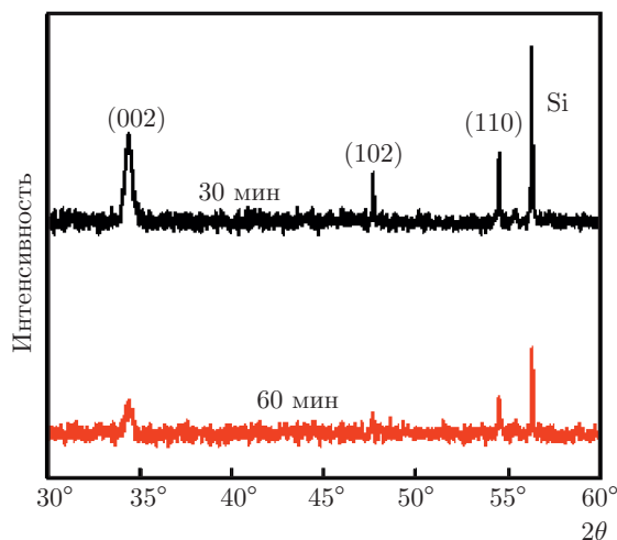
Рис. 1. Рентгенограммы пленок ZnO, отожженных при температуре 300^\circ\text{C} в течение 30 и 60 мин в потоке кислорода 20 \text{ см}^3/\text{мин}
