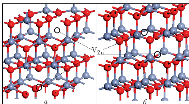
Рис. 5. (В цвете онлайн) Сверхячейка с двумя вакансиями цинка: а — две изолированные вакансии; б — две близкие вакансии
