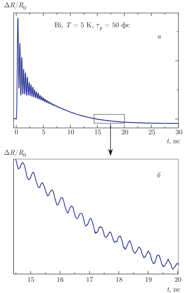
Рис. 14. (В цвете онлайн) а) Зависимость дифференциального отражения \Delta R/R_0 от времени для монокристалла Вi при гелиевой температуре в нелинейном режиме возбуждения. Длительность импульса возбуждения 70 фс. б) Увеличенный сигнал для обозначенного прямоугольником временного окна на панели а
