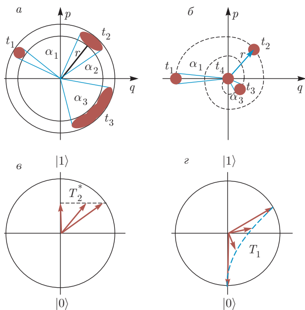
Рис. 1. (В цвете онлайн) Схематическая иллюстрация чистой дефазировки ( a , e ) и энергетической релаксации ( б , з ) КФ при их классическом ( a , б ) и квантовомеханическом ( e , з ) представлениях. На нижних панелях приведено схематическое сечение сферы Блоха, полюса которой соответствуют вакуумному |0\rangle и однофононному |1\rangle состояниям, и демпфирующие процессы в блоховском представлении. Процессы поперечной релаксации ( e ), ответственные за T_2^* , сохраняют z -компоненту вектора Блоха r^2 = x^2 + y^2 + z^2 , а процессы продольной релаксации ( з ), контролируемые T_1 , приводят к изменению z -компоненты вектора
