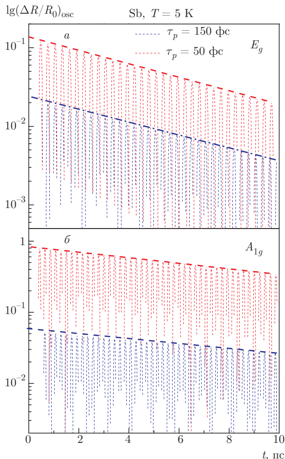
Рис. 6. (В цвете онлайн) Осциллирующие вклады отражения различной симметрии (а — E_g , б — A_{1g} ) сурьмы, полученные при различных длительностях импульса накачки, в полулогарифмических координатах. Штриховые линии позволяют сравнить времена жизни КФ, которые практически совпадают для больших и малых когерентных амплитуд, реализованных при помощи изменения длительности импульса возбуждения
