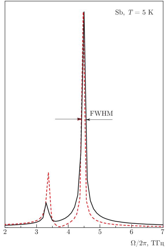
Рис. 4. (В цвете онлайн) Нормированные фурье-образы осциллирующего вклада отражения Sb при T = 5 K для двух различных длительностей импульса возбуждения: \tau_p = 150 фс (штриховая кривая) и \tau_p = 50 фс (сплошная кривая)
