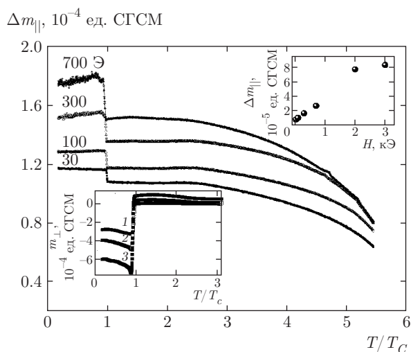
Рис. 4. Температурные зависимости магнитного момента m_{\parallel} для гетероструктуры № 1 при охлаждении в магнитных полях (режим FC) для H = 30, 100, 300, 700 Э. Переход пленки SRO в ферромагнитное состояние наблюдается при T/T_C = 2.5 . Вставка внизу: зависимости величин магнитного момента m_{\perp} в поле, перпендикулярном плоскости подложки, измеренные в полях: 1 — 30, 2 — 200, 3 — 500 Э. На вставке сверху представлена зависимость изменения магнитного момента \Delta m_{\parallel} гетероструктуры от величины внешнего магнитного поля при T \approx T_C
